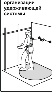
Рис. 12. Способ организации удерживающей системы
