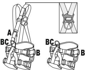
Рис. 12. Позиционирование в рабочем положении
