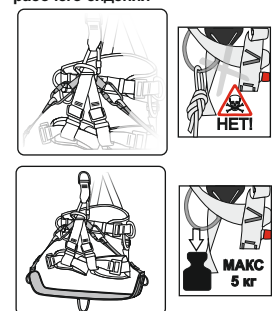
Рис. 14. Способ интеграции рабочего сидения
