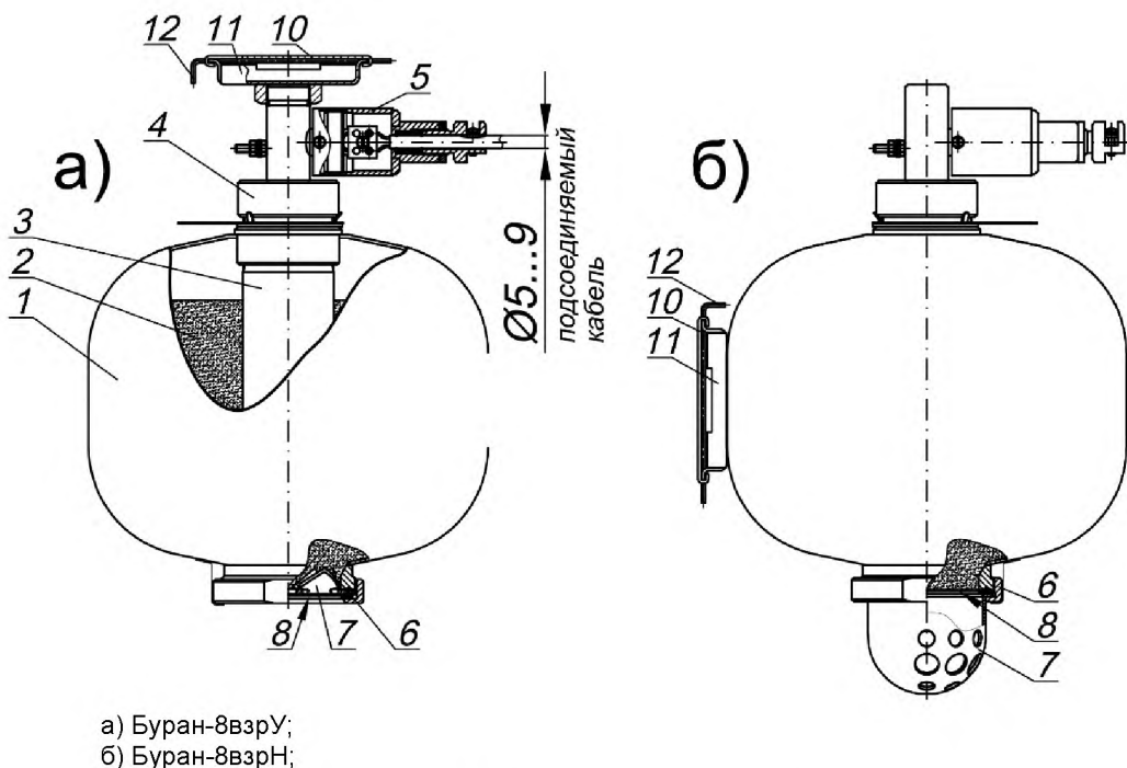
Рис. 1 - Устройство модуля.
