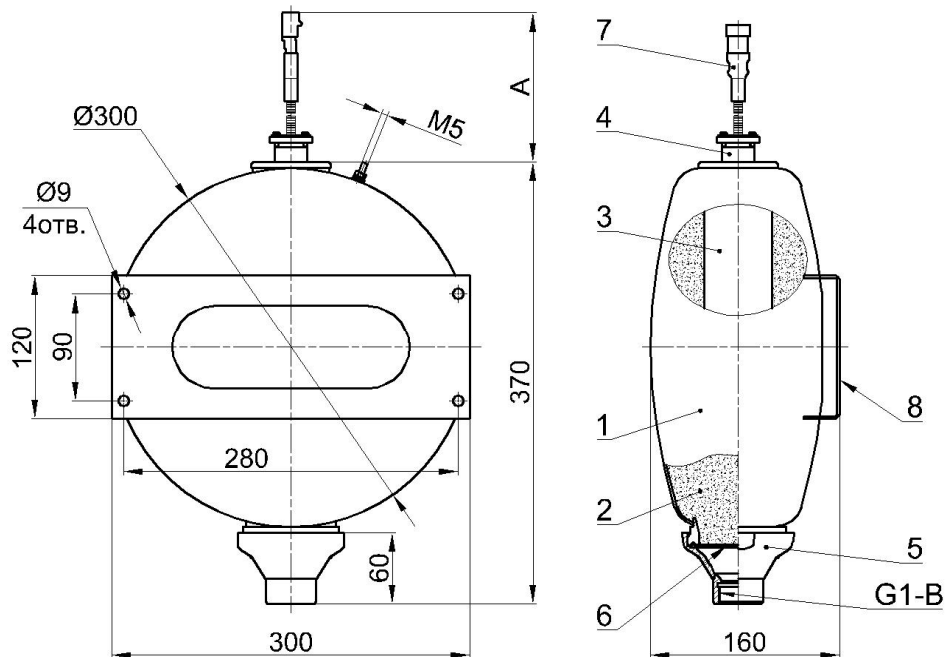
Рисунок 1.2 – Устройство и габаритные размеры модуля Буран-7КДТН
