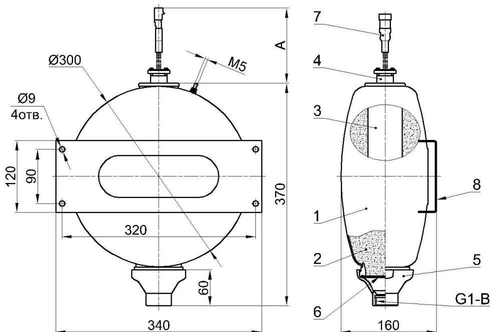
Рисунок 1.3 – Устройство и габаритные размеры модуля Буран-7КДТН(340) с удлиненным кронштейном.
