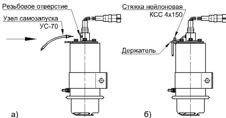
Рисунок 1 – Замена узла самозапуска.
